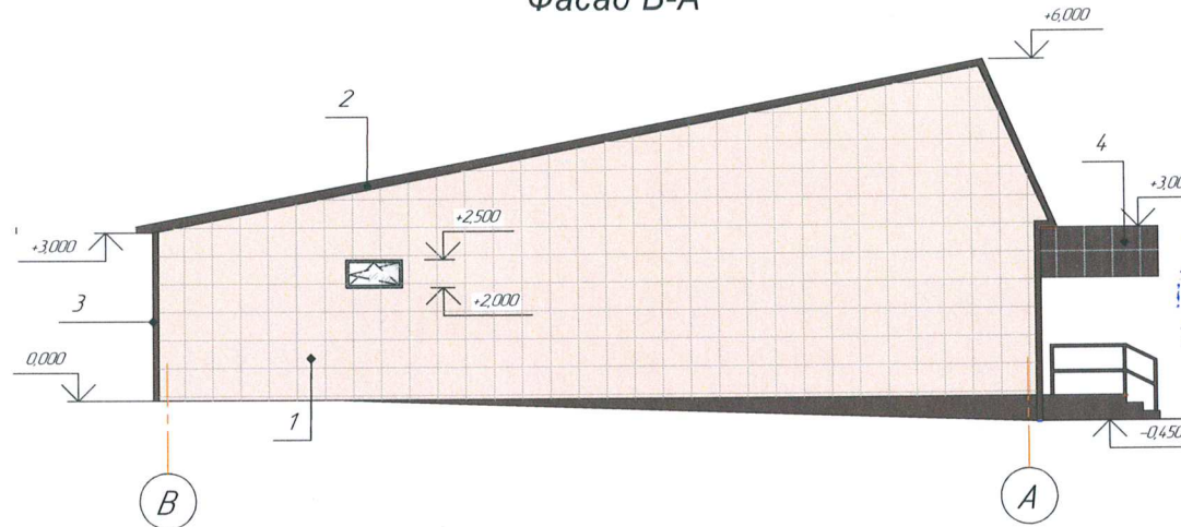
Фасад В-А
