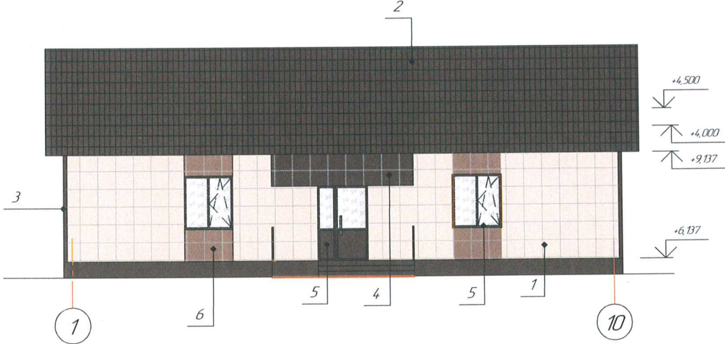
Фасад 1-10
